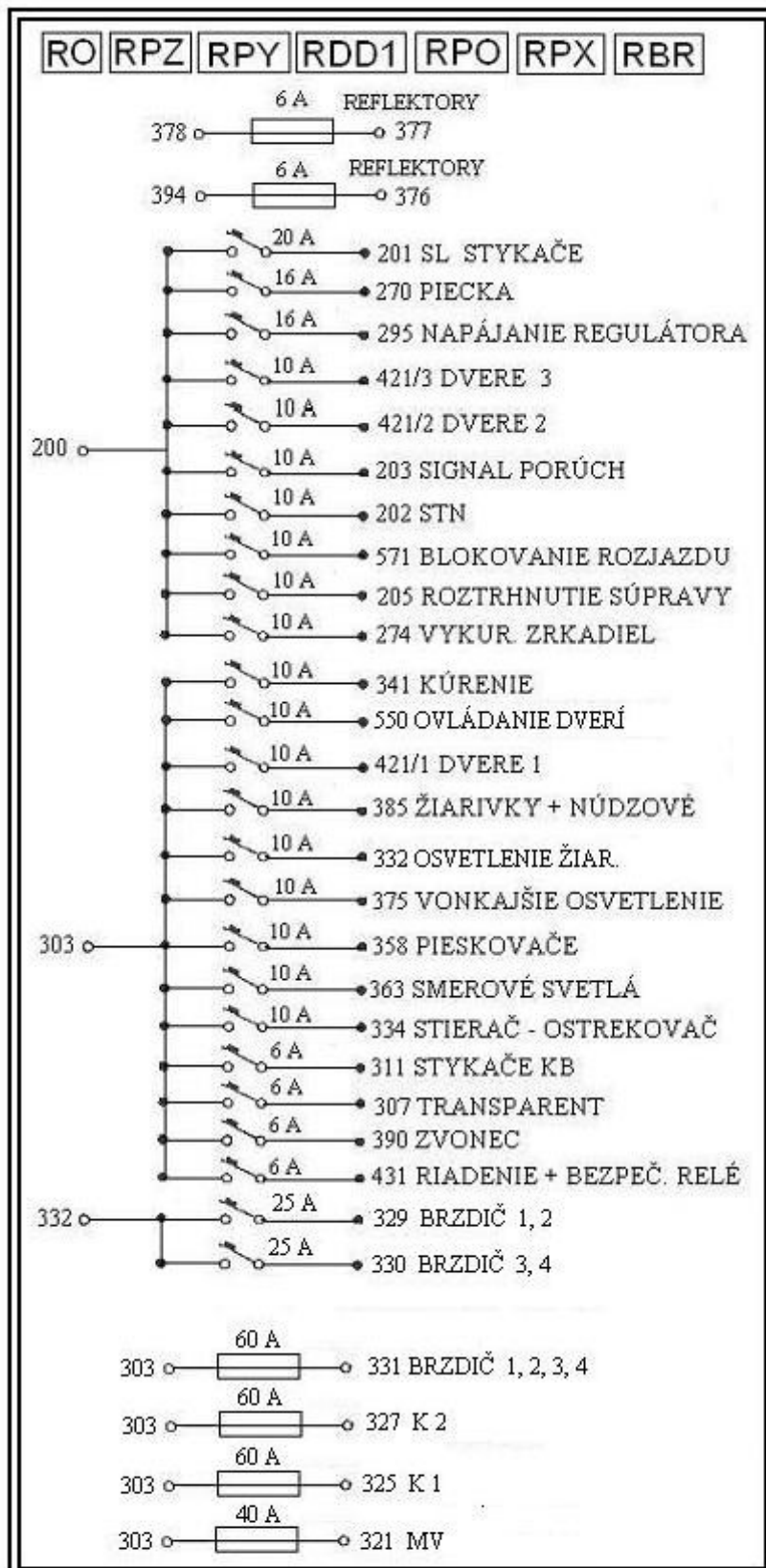
T6A5 - ISTIČE A POISTKY
